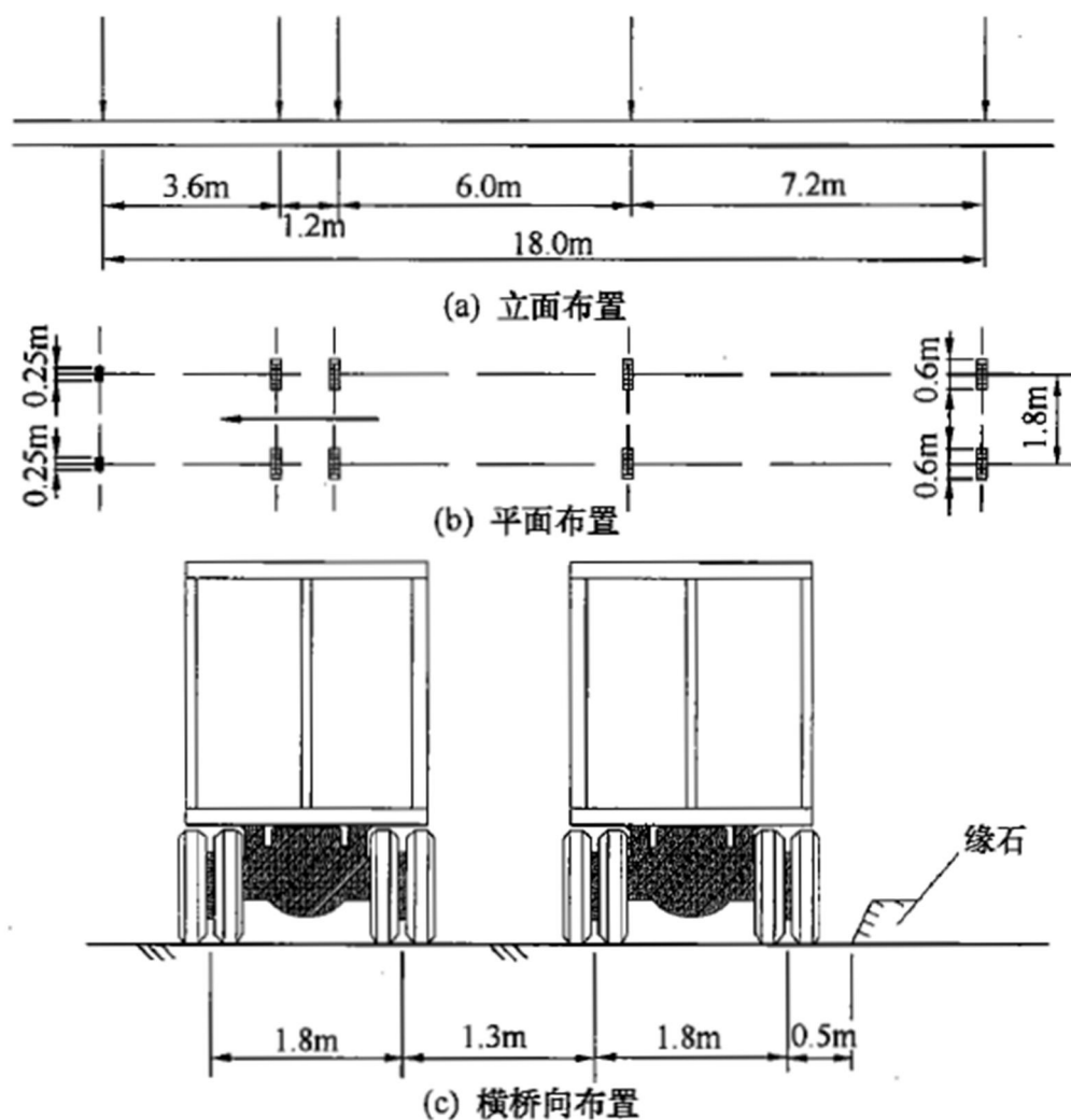
图 10.0.2-2 城 -A级车辆荷载立面、平面、横桥向布置
