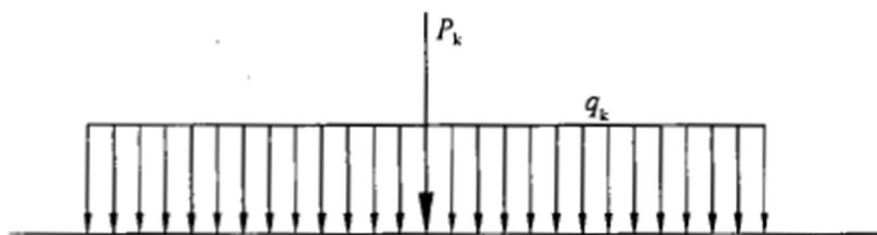
图 10.0.2-1 车道荷载
